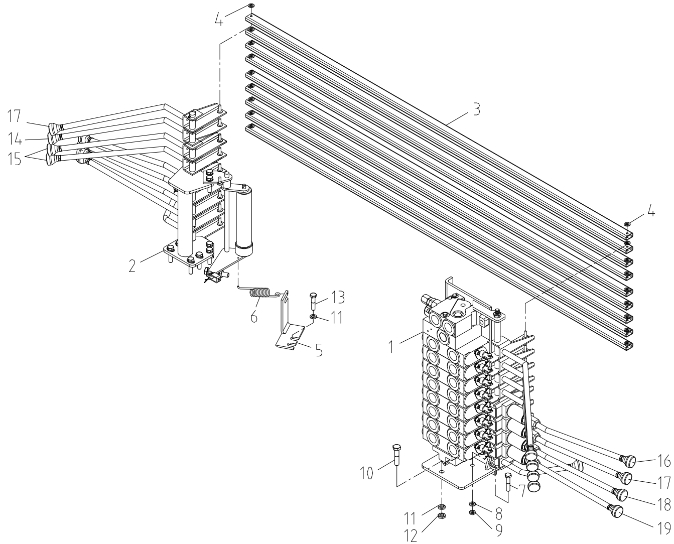
오퍼레이션 메인 조립체 Fig. 3-4 SCS514SL OPERATION MAIN ASS'Y
