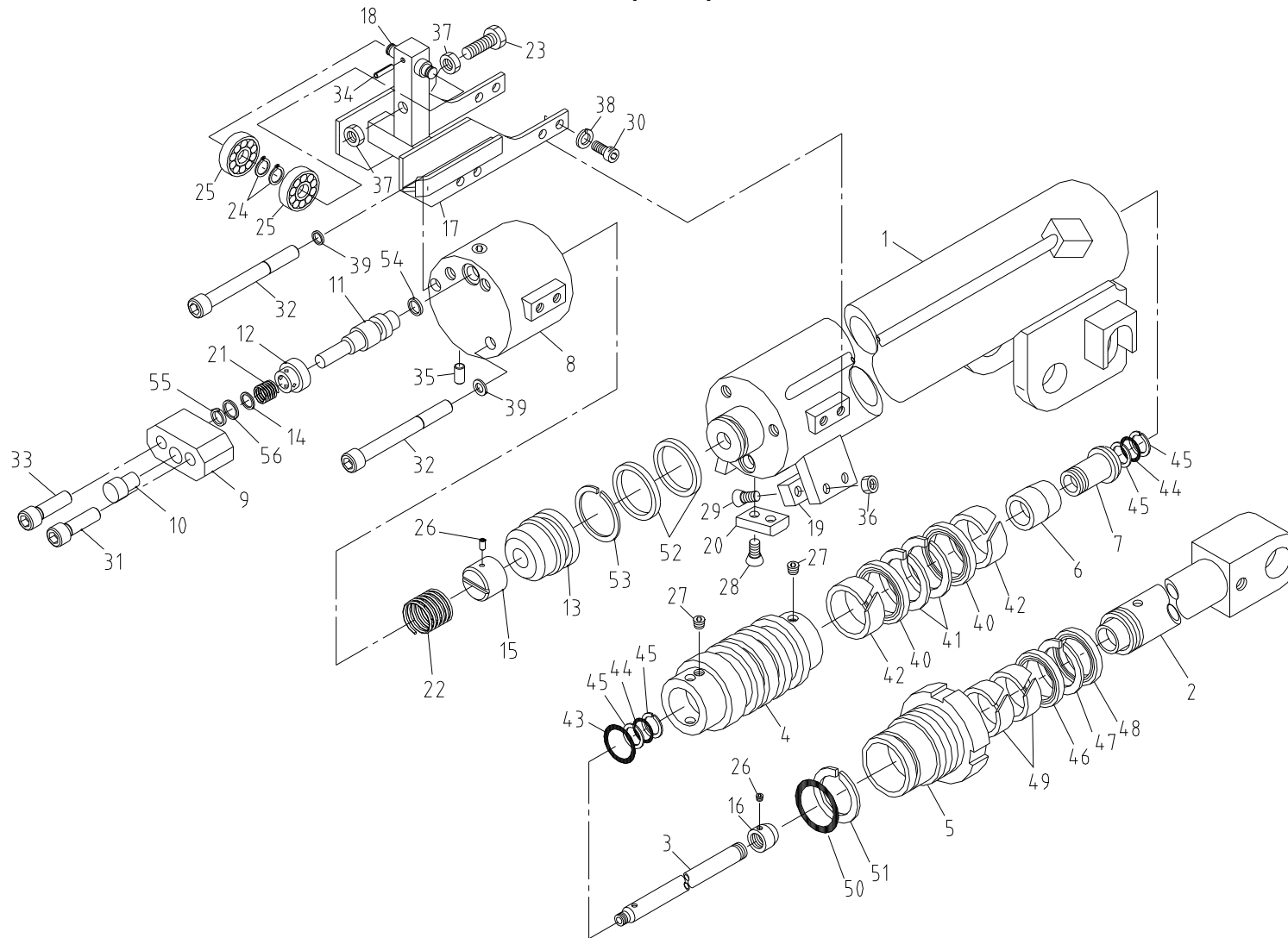
텔레스코픽 실린더(2단) 조립체 Fig. 1-1-2 SCS514SL TELESCOPIC CYL'(2nd) ASS'Y
