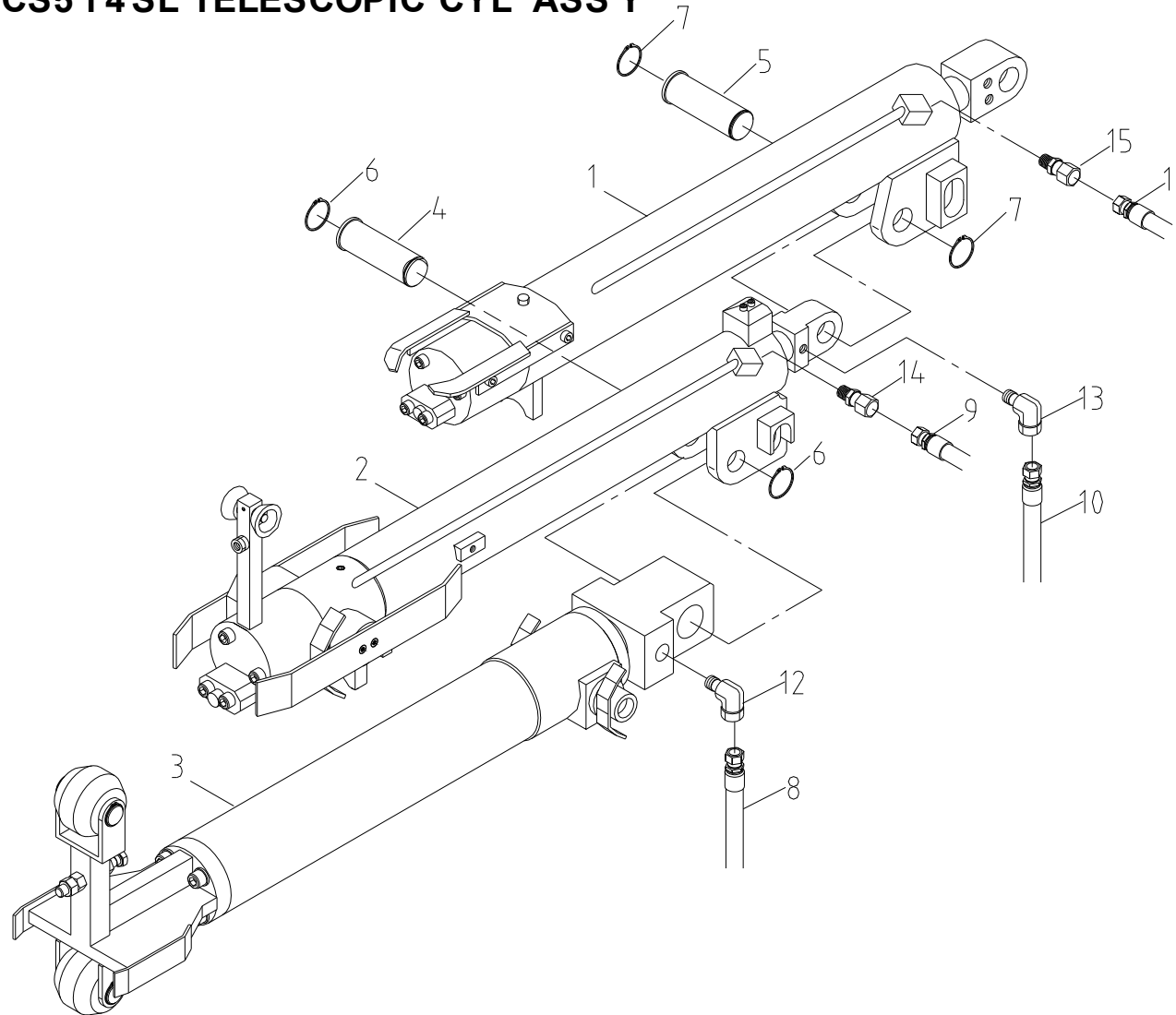
텔레스코픽 실린더 조립체 Fig. 1-1 SCS514SL TELESCOPIC CYL' ASS'Y
