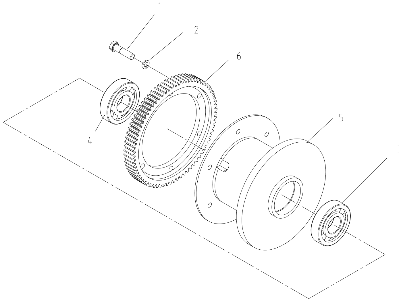
드럼 조립체 Fig. 2-1 SCS514SL DRUM ASS'Y
