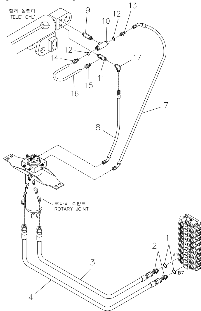
텔레스코픽 배관 Fig. 5-4 SCS514SL TELESCOPIC PIPING
