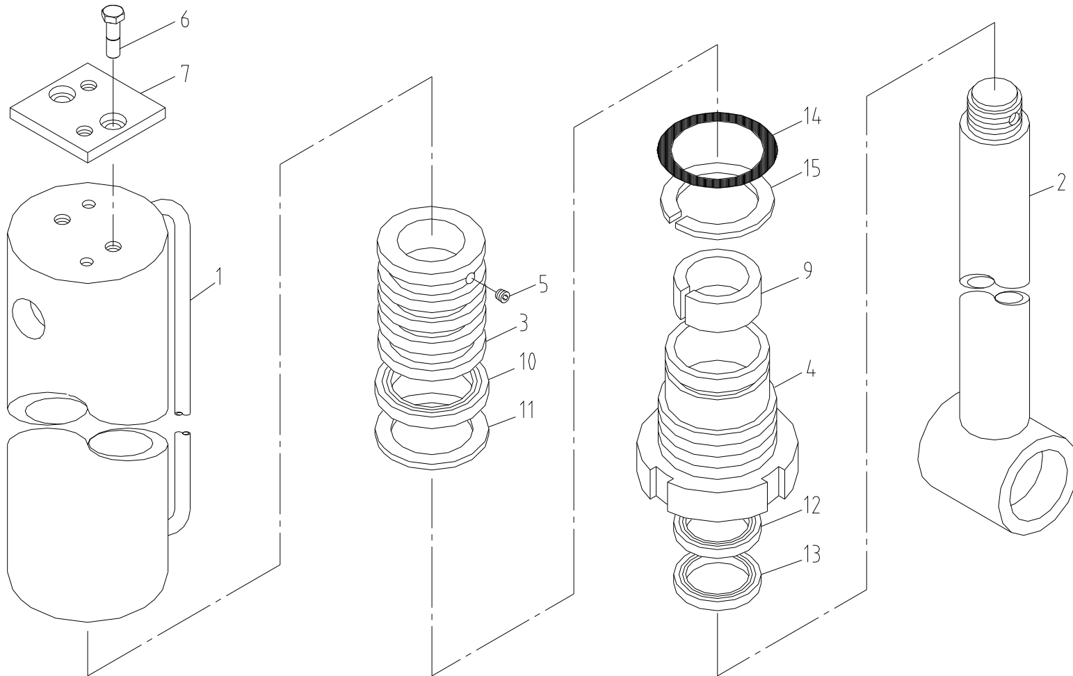
잭 실린더 조립체 Fig. 4-1 SCS514SL JACK CYL' ASS'Y
