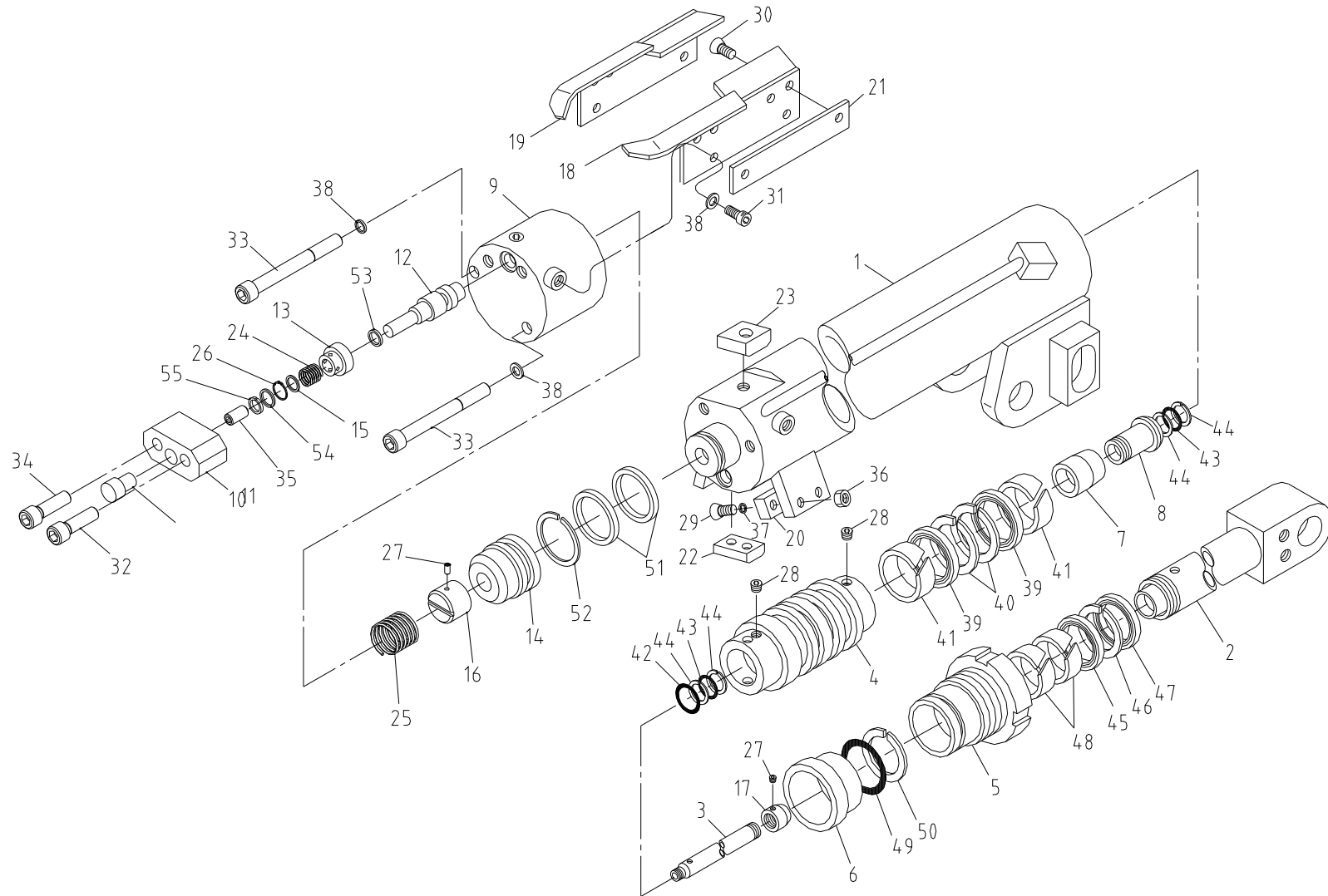
텔레스코픽 실린더(1단) 조립체 Fig. 1-1-1 SCS514SL TELESCOPIC CYL'(1st) ASS'Y
