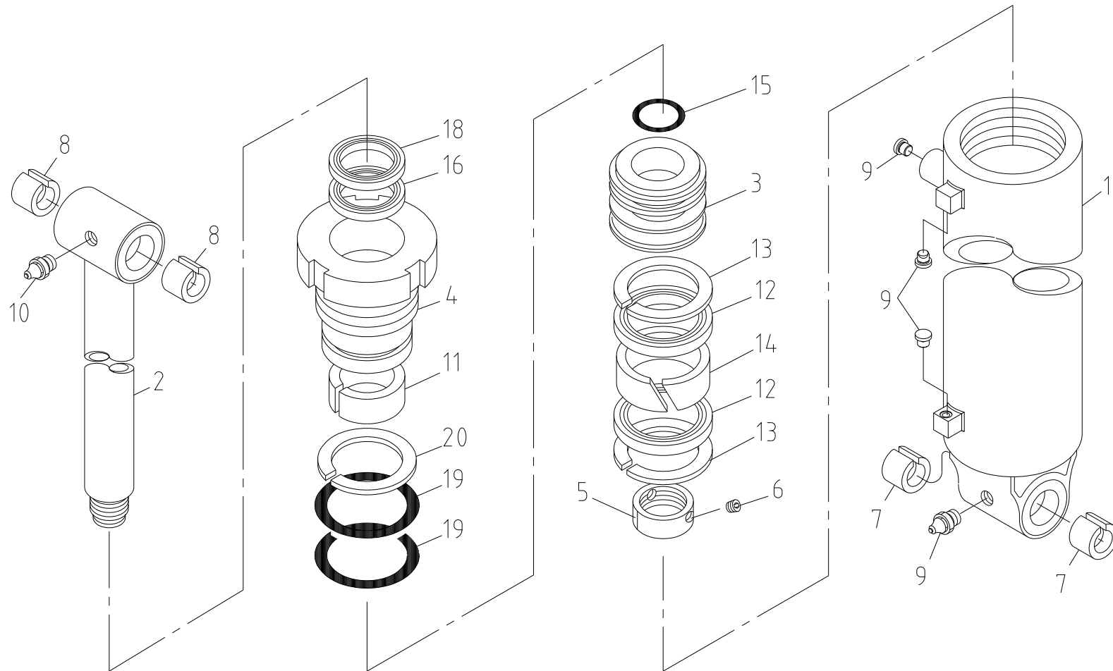
데릭 실린더 조립체 Fig. 2-3 SCS514SL DERRICK CYLINDER ASS'Y
