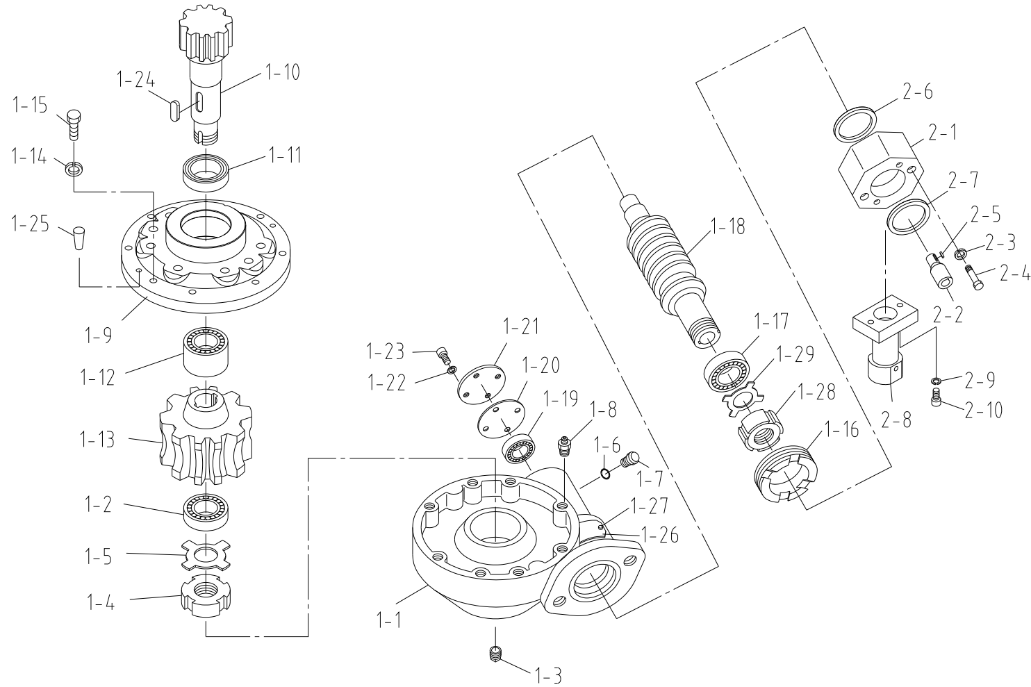
스윙 감속기 세트 Fig. 3-1 SCS514SL SWING R/ G SET
