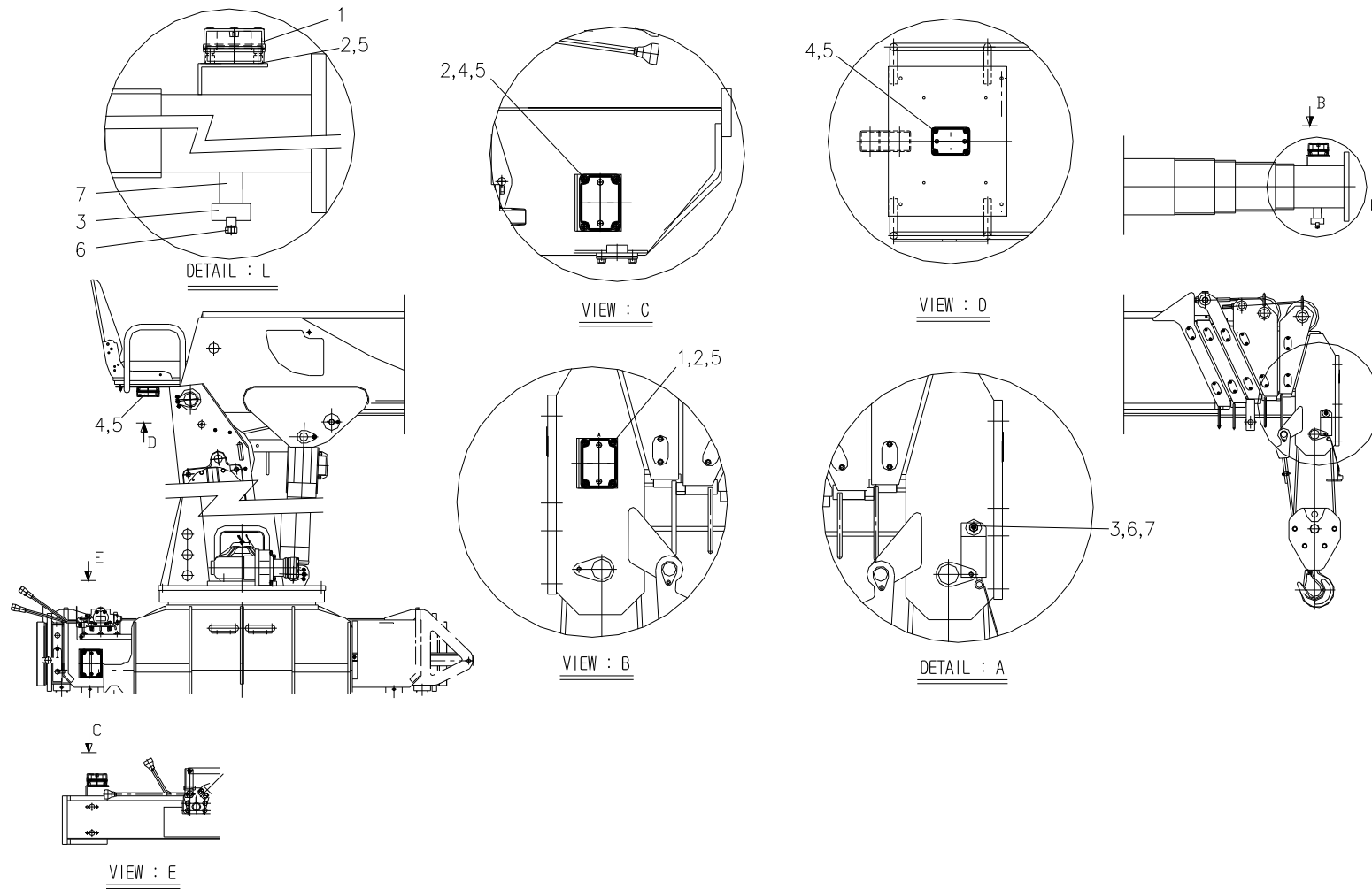
Fig. 9-3-1 SCS514SL 무선 과관 장치 위치도
